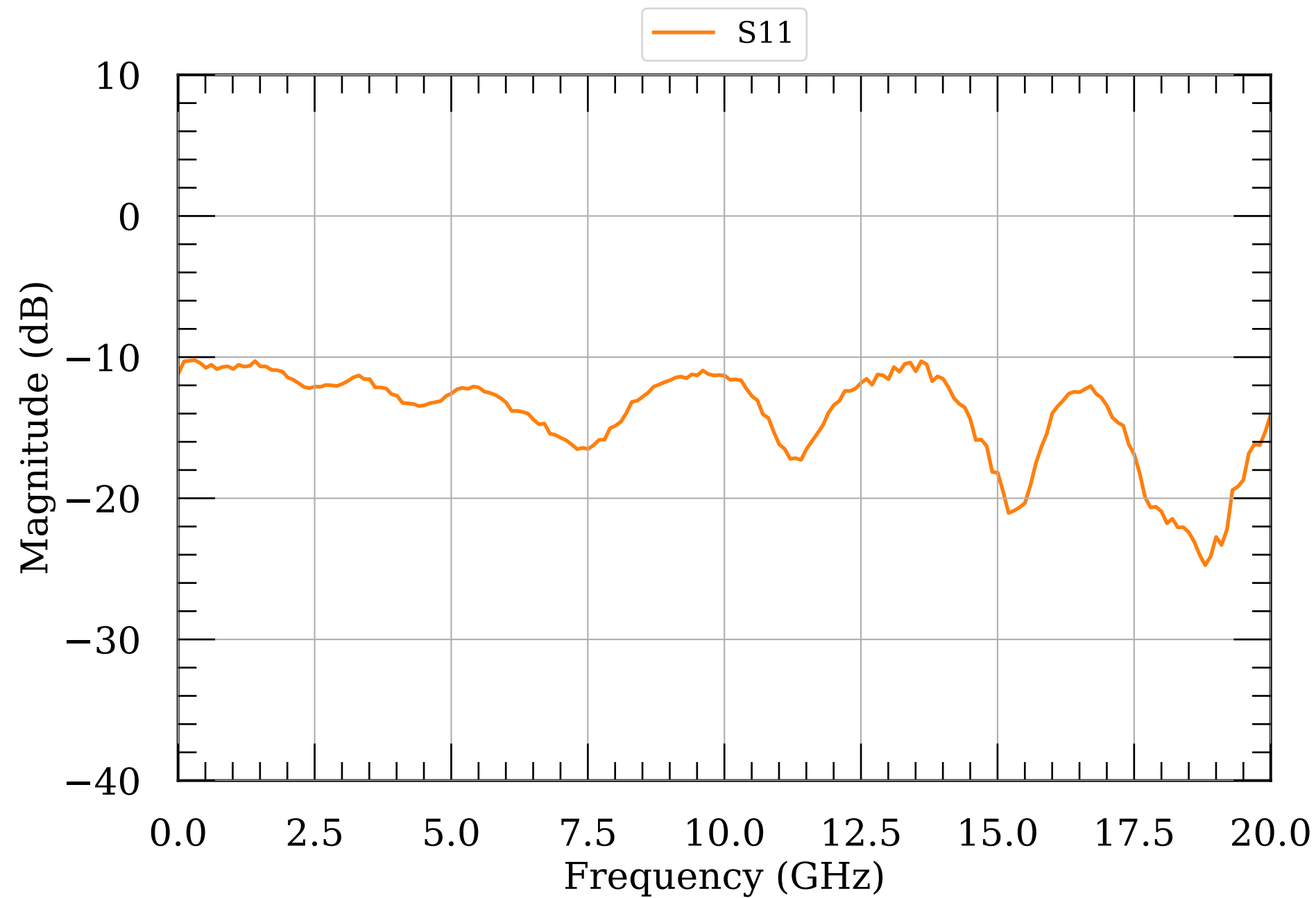
LNA S-params module071
